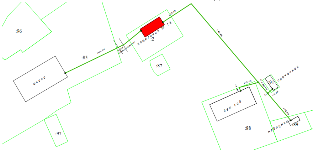
Рис.1.4.5 – Зона действия котельной №16 д. Захарвань
