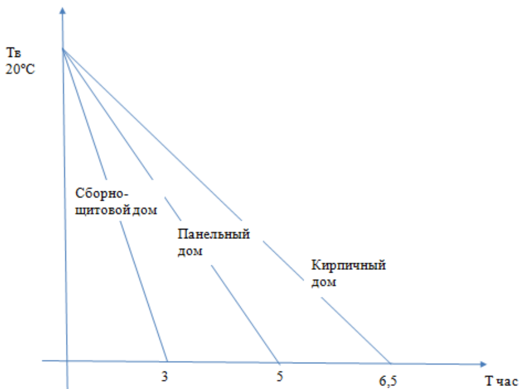
Рисунок 11.1 – График снижения температуры воздуха в отопляемых помещениях здания при отключении системы отопления для панельных, кирпичных и сборно-щитовых домов при температуре наружного воздуха -40^{\circ}\text{C} .
